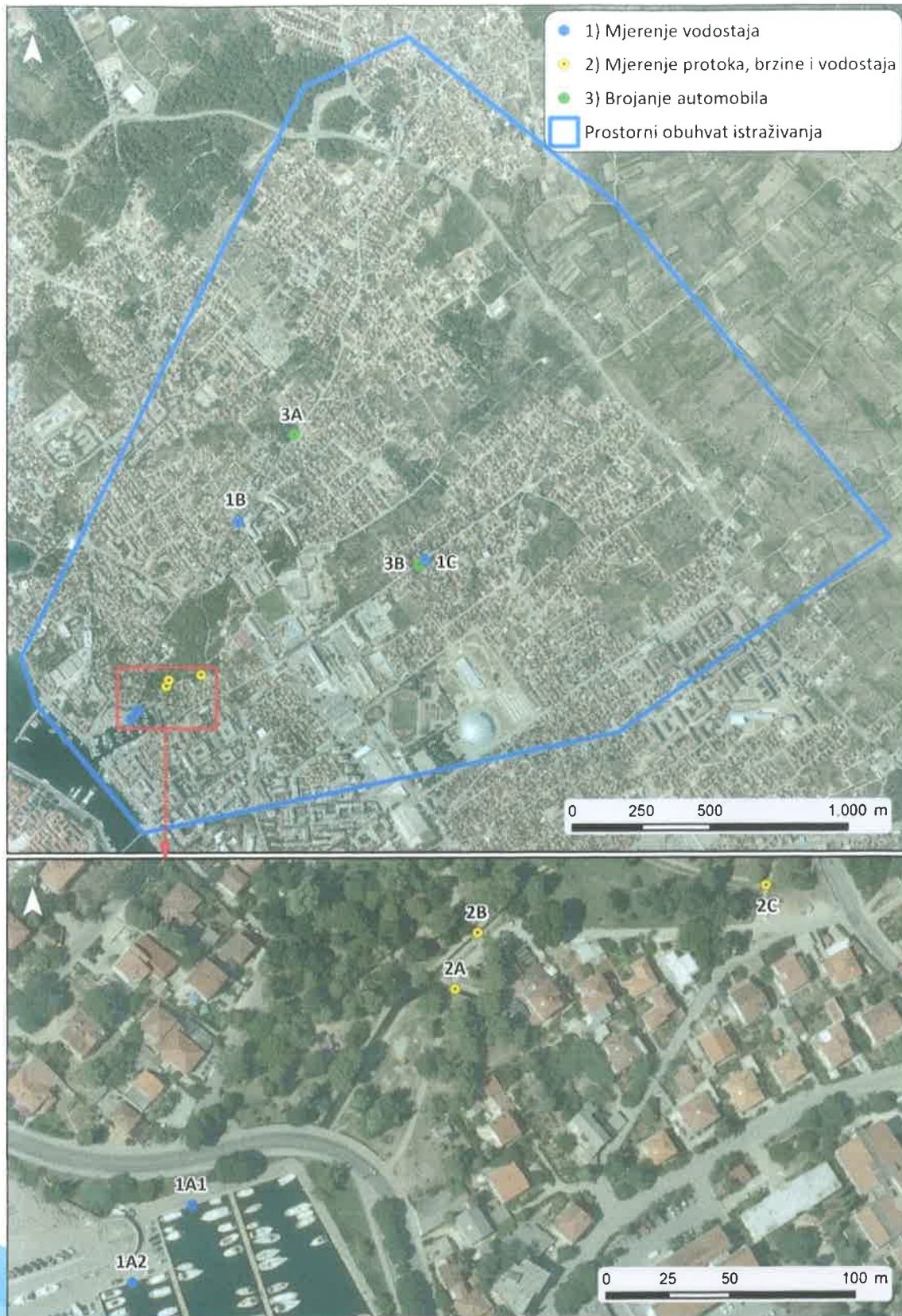
Slika 5. Oznake potencijalnih lokacija za ugradnju senzora za mjerenje protoka, brzine, vodostaja i brojanje automobila
