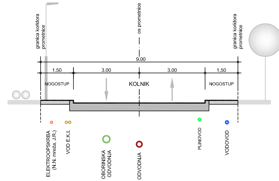
KARAKTERISTIČAN PROFIL PROMETNICE A-A (9.00 m) M 1:100
