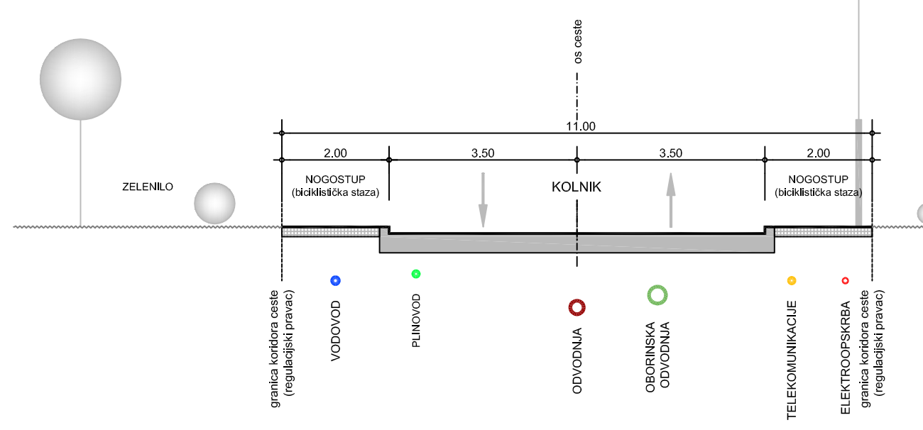
KARAKTERISTIČAN PROFIL PROMETNICA 3-3 I 4-4 (11,00 m)
