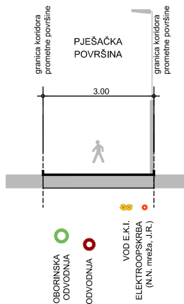
KARAKTERISTIČAN PROFIL PJEŠAČKOG KORIDORA C-C (3.0 m)
