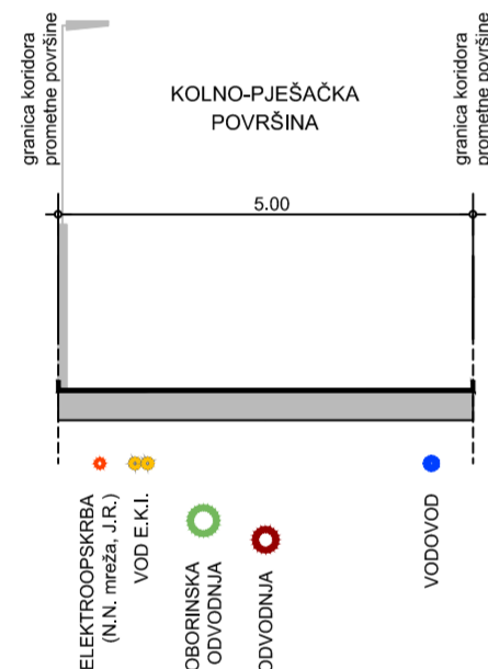
KARAKTERISTIČAN PROFIL KOLNO-PJEŠAČKE POVRŠINE B-B (5.0 m)
