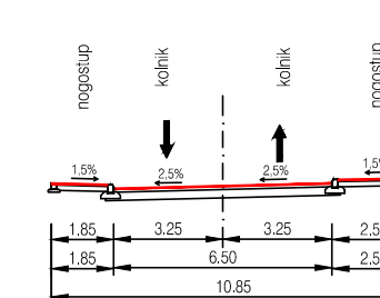
PRESJEK B - B
