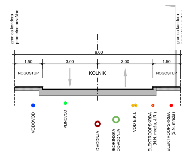
KARAKTERISTIČAN PROFIL CESTE A-A (9.0 m)
