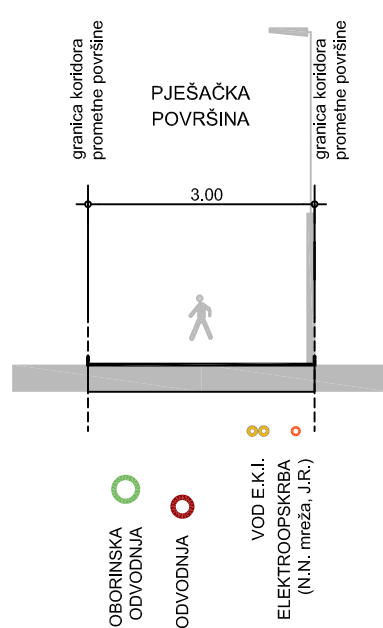
KARAKTERISTIČAN PROFIL PJEŠAČKOG KORIDORA C-C (3.0 m)
