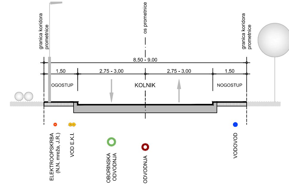
KARAKTERISTIČAN PROFIL PROMETNICA A-A (9.00 m), B-B (8.50 m)
