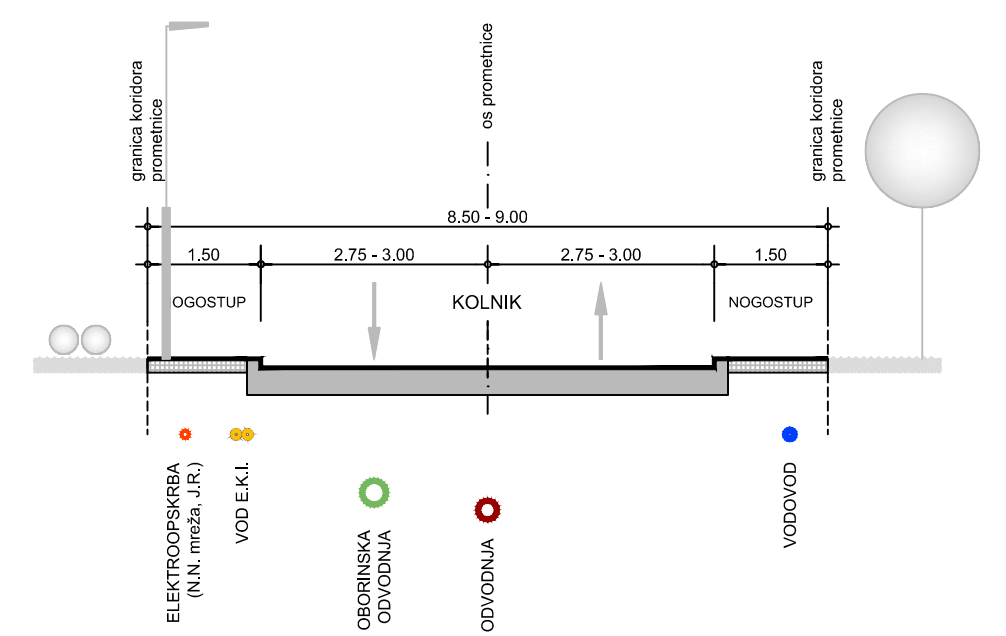
KARAKTERISTIČAN PROFIL PROMETNICA A-A (9.00 m), B-B (8.50 m) M 1:100
