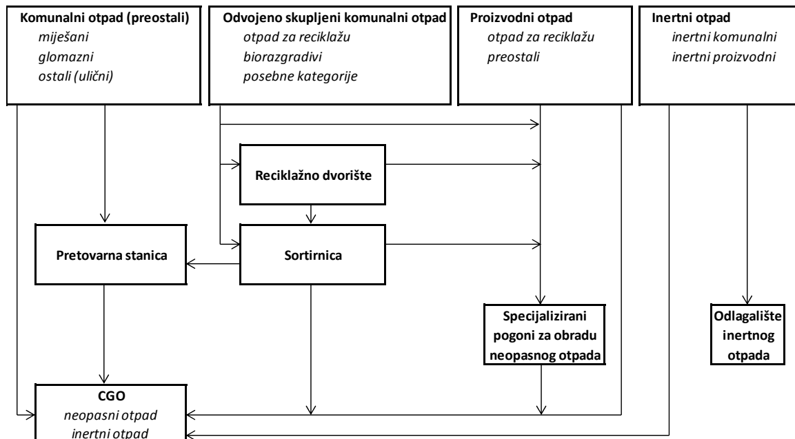
Slika 3.2-1/2: Shema gospodarenja neopasnim i inertnim otpadom
