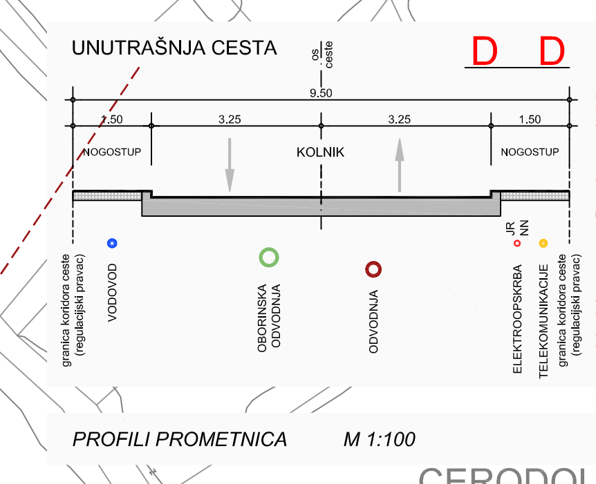
PROFILI PROMETNICA M 1:100
