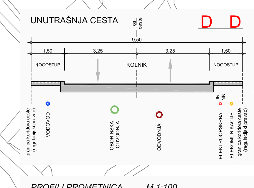
PROFILI PROMETNICA M 1:100
