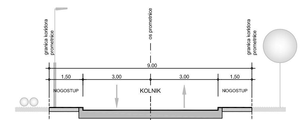
KARAKTERISTIČAN PROFIL PROMETNICE A-A (9.00 m) M 1:100
