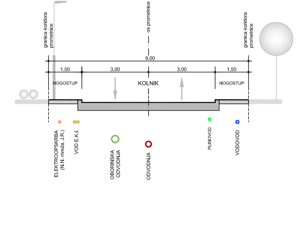
KARAKTERISTIČAN PROFIL PROMETNICE A-A (9.00 m) M 1:100
