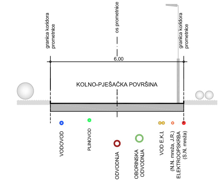
KARAKTERISTIČAN PROFIL PROMETNICE B-B (6.00 m) M 1:100
