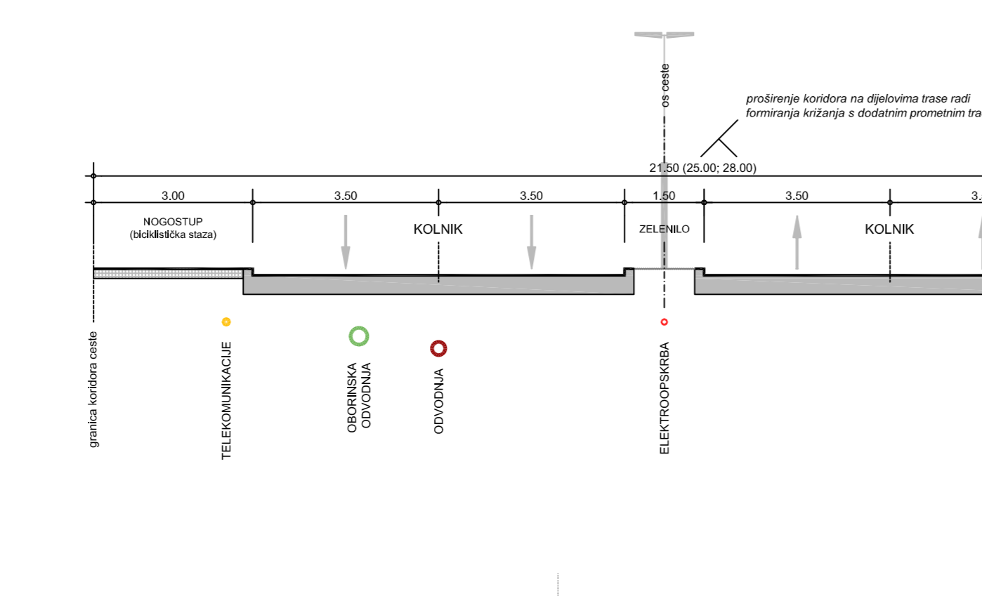
KARAKTERISTIČAN PROFIL PROMETNICE 3-3 (21.50 m) M 1:100
