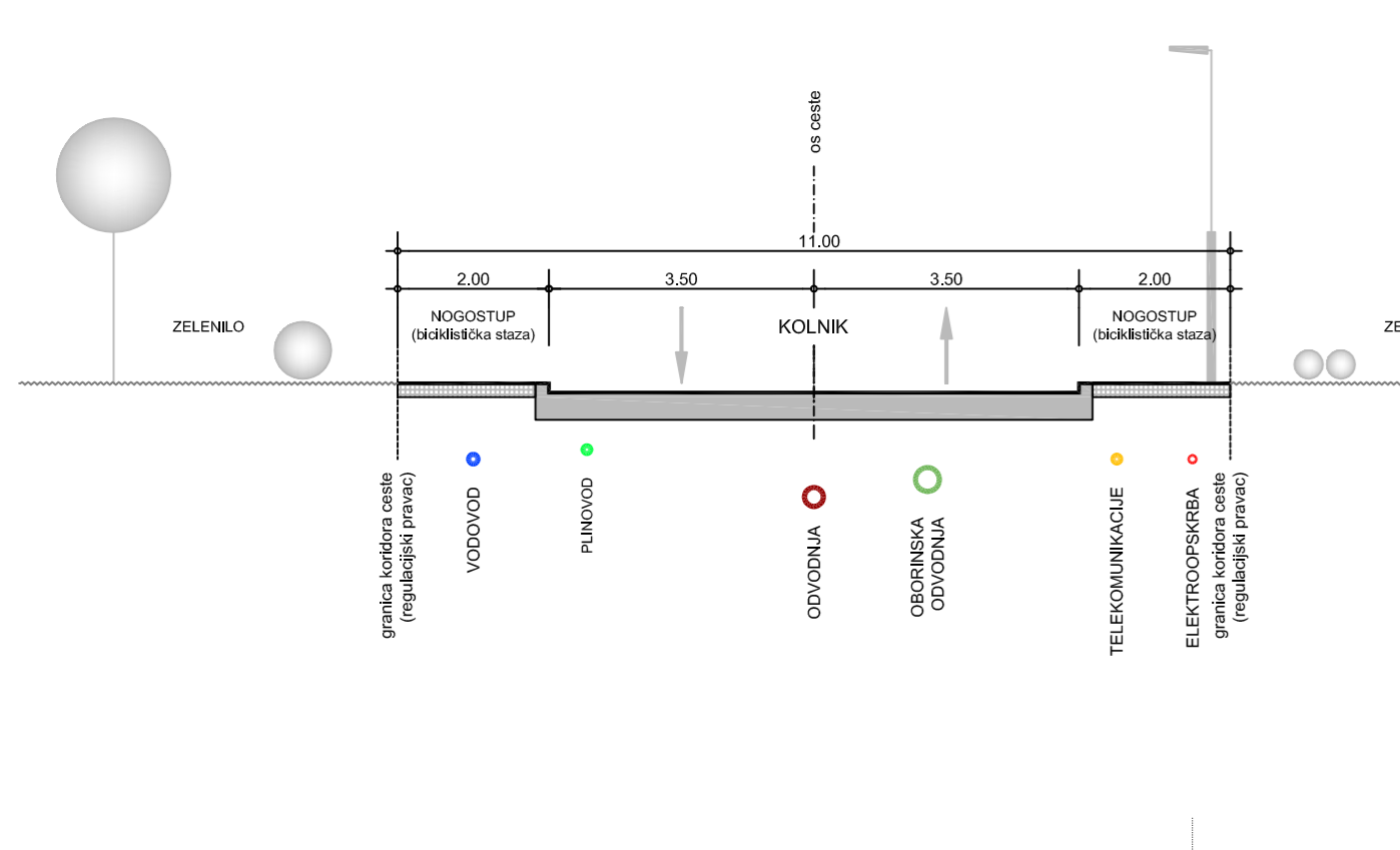
KARAKTERISTIČAN PROFIL PROMETNICA 4-4 (11.00 m) M 1:100
