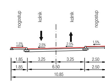
PRESJEK B-B
