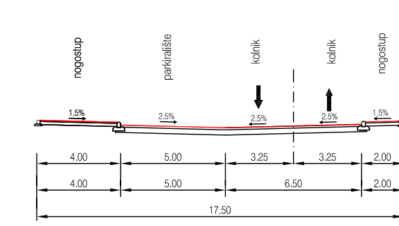
PRESJEK D-D
