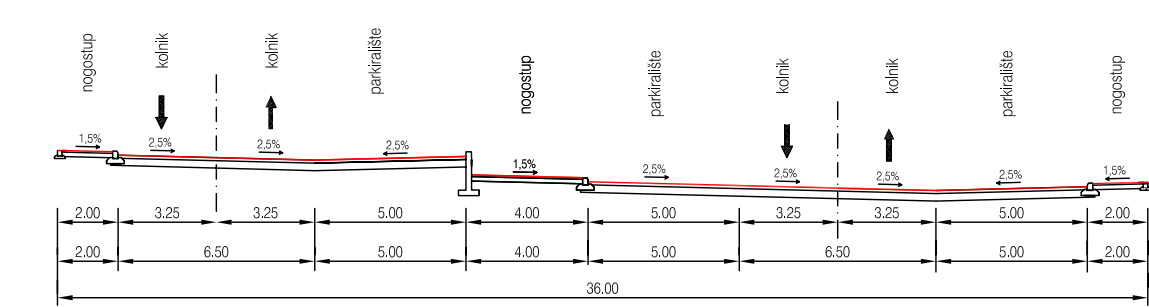
PRESJEK C-C
