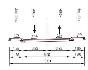
PRESJEK A-A
