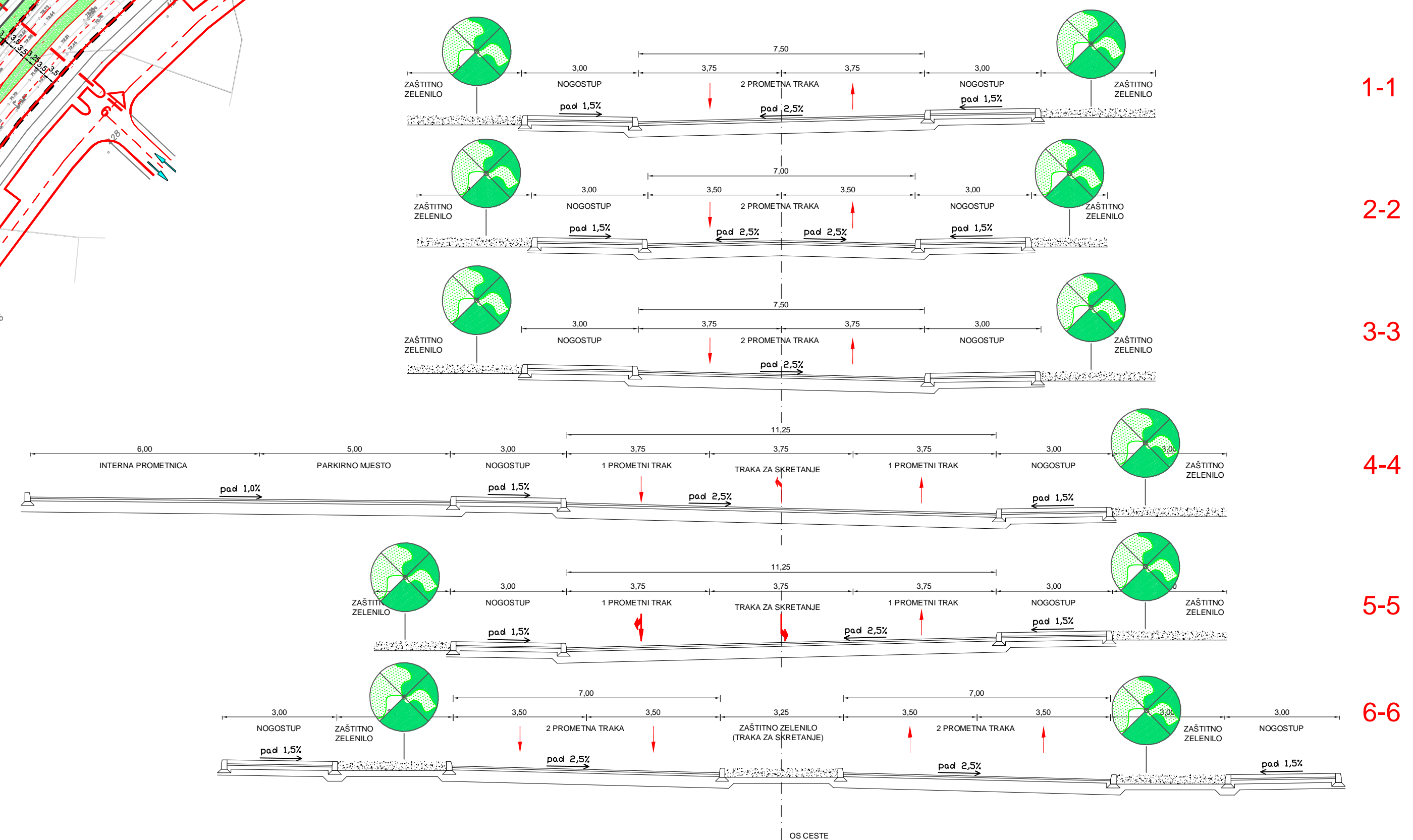
karakteristicni presjeci mj 1:100
