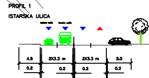
POPREĀNI PROFILI PROMETNICA
