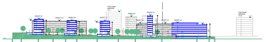
PRESJEK B-B
