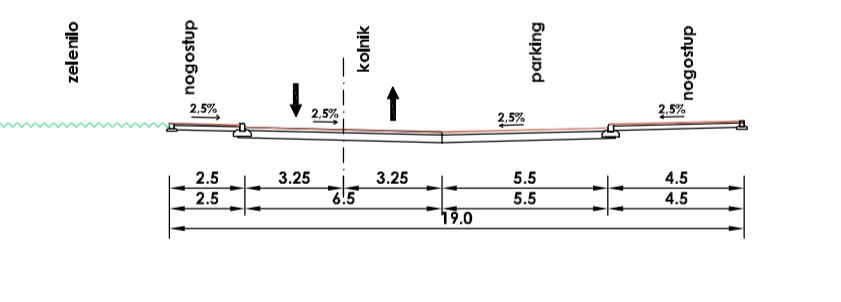
F - F UNUTRAŠNJA ULICA
