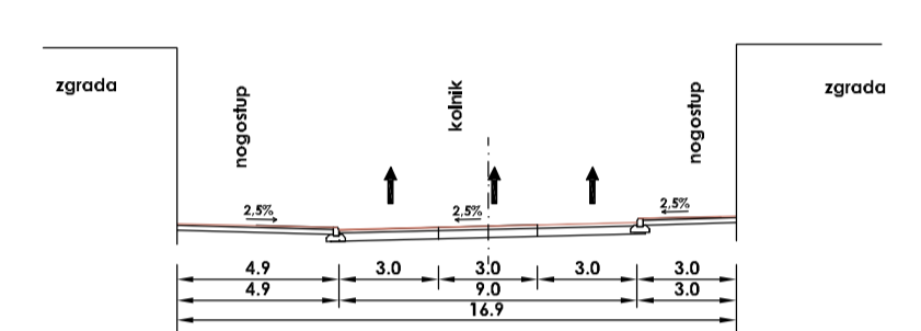
C - C ULICA ZRINSKO-FRANKOPANSKA
