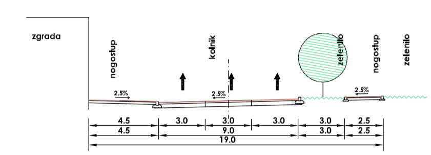
B - B ULICA LJ. POSAVSKOG
