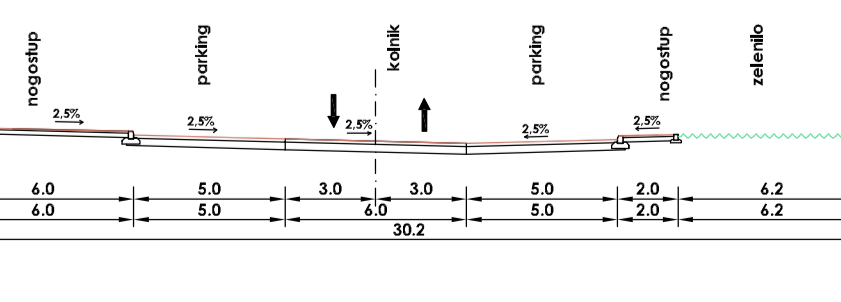
H - H UNUTRAŠNJA ULICA
