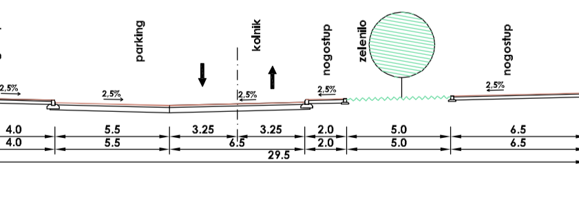
G - G UNUTRAŠNJA ULICA
