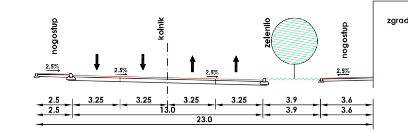
A - A ULICA N. Š. ZRINSKOG
