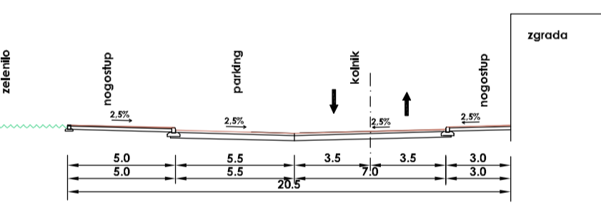
E - E ULICA E. KVATERNIKA
