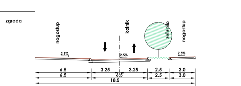
D - D ULICA ZRINSKO-FRANKOPANSKA
