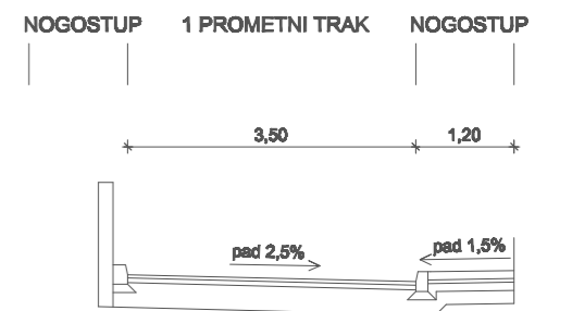
PRESJEK 2-2, MJ 1:100
