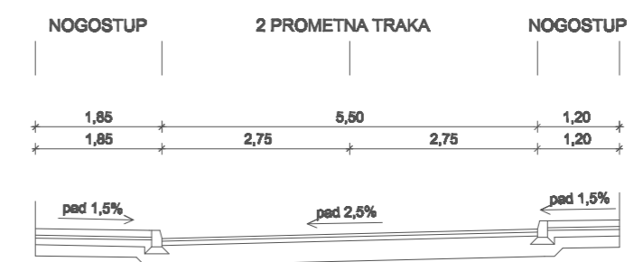
PRESJEK 1-1, MJ 1:100
