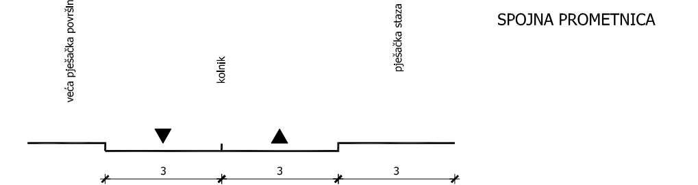
PRESJEK 5 SPOJNA PROMETNICA
