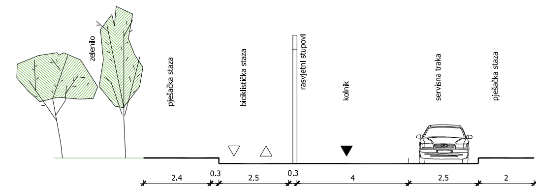
PRESJEK 2 OBALA KNEZA TRPIMIRA
