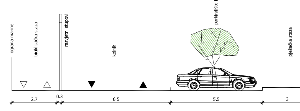
PRESJEK 3 OBALA KNEZA TRPIMIRA
