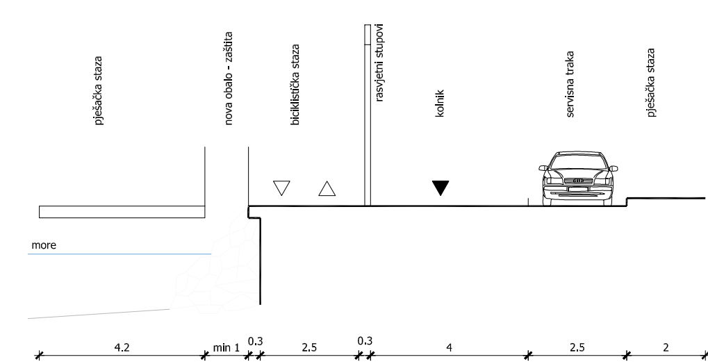
PRESJEK 1 OBALA KNEZA TRPIMIRA
